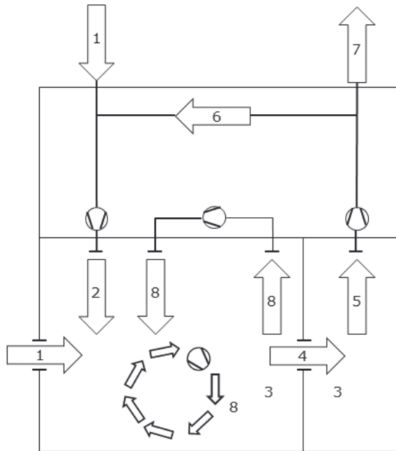
Kuva 1.1 Ilmavirtojen nimet ja määritelmät. Kuva on osittainen kopio standardin SFS-EN 16798-3:2017 standardista. Kuvaan on merkitty vain asetustekstin määritelmässä mainitut ilmavirrat.
