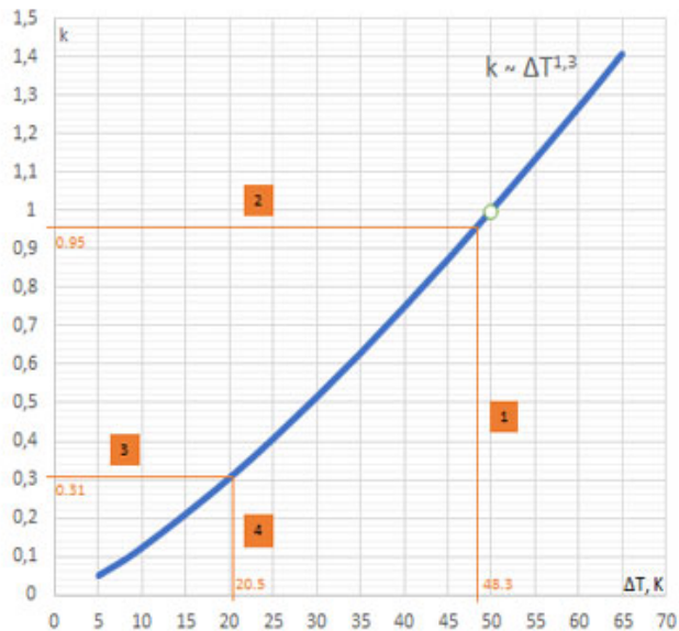
Kuva 3. Radiaattorin tehosuhteen k riippuvuus yllilämpötilasta T .
