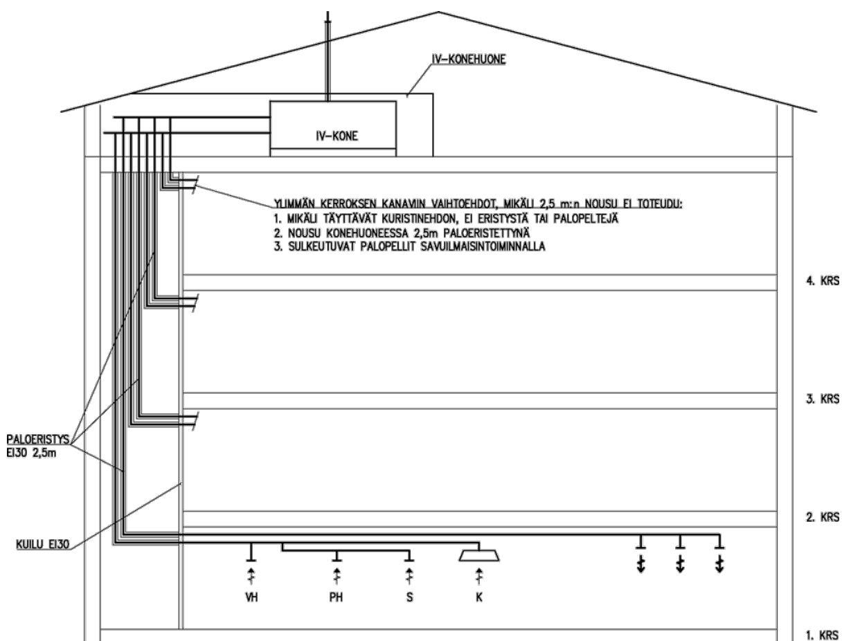
Kuva 7.5b Keskusilmanvaihtokoneella ja eristetyillä asuntokohtaisilla nousukanavilla toteutettu asuntoilmanvaihdon ratkaisu.
