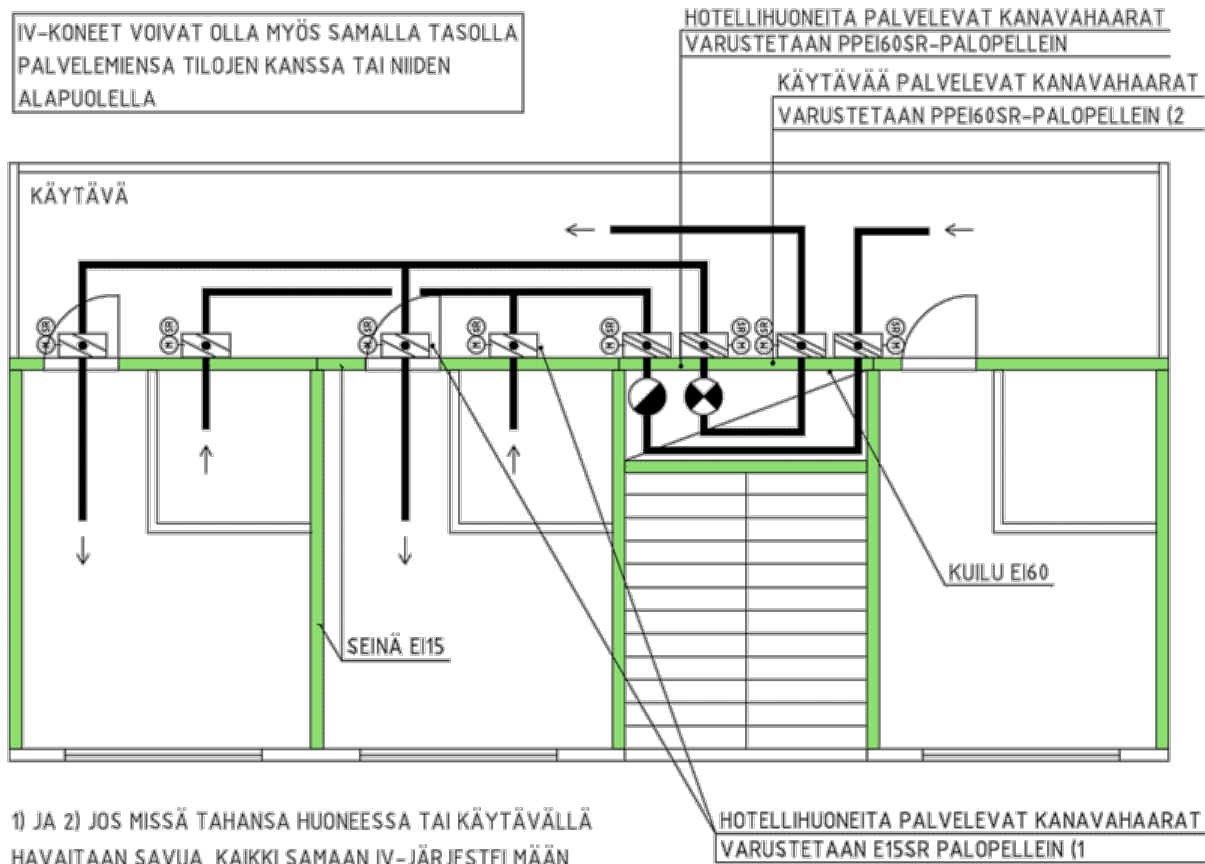
Kuva 7.7b IV-koneet voivat olla myös palvelemiensa tilojen alapuolella.
