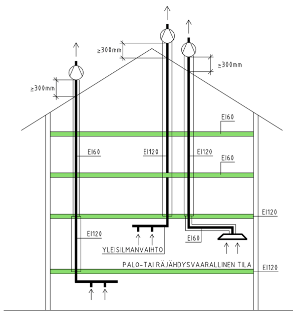
Kuva 9.2. Palo- ja räjähdysvaarallisen tilan ilmanakanavien palonkestävyys.
