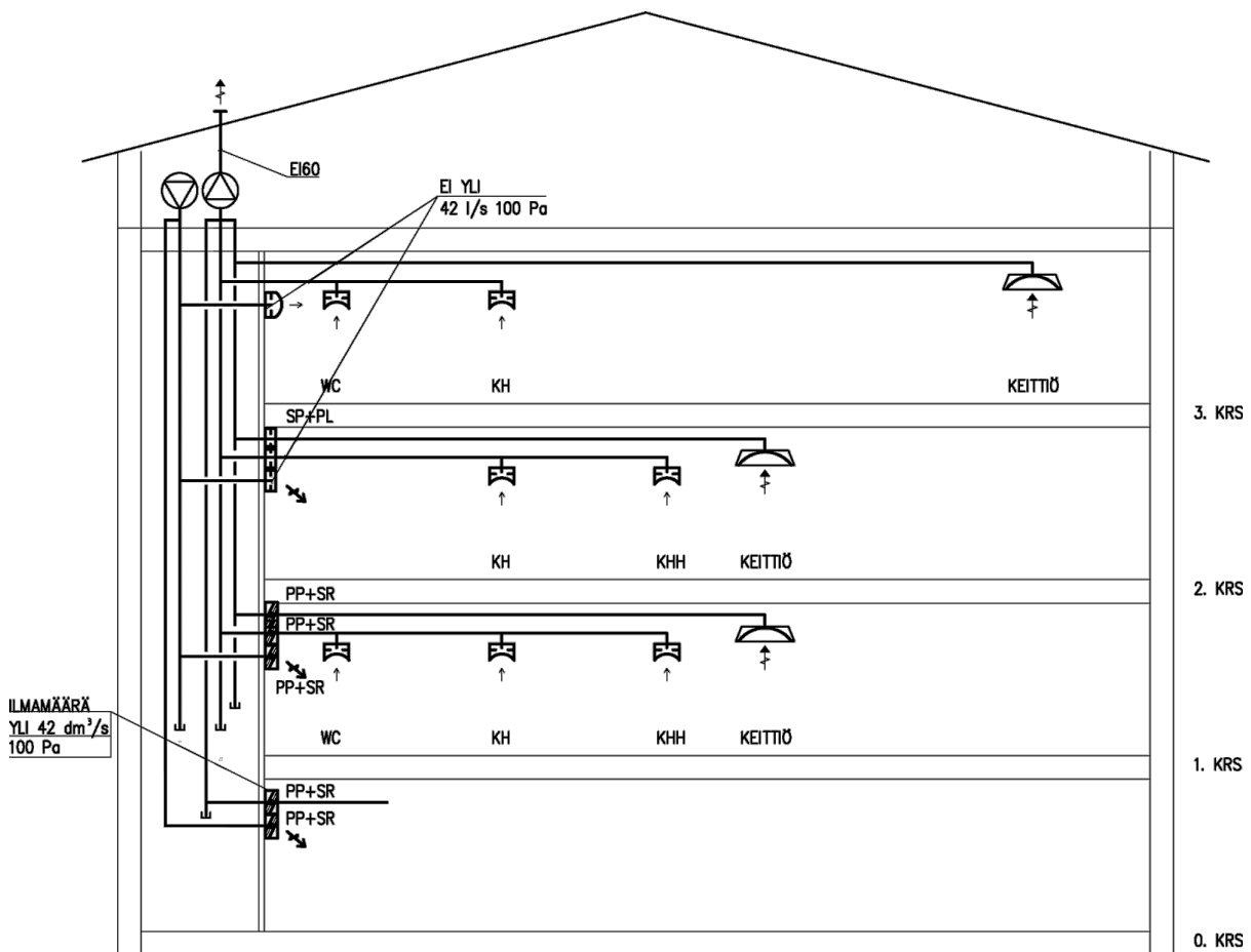
Kuva 7.5 Esimerkki asuinkerrostalon keskitetystä ilmanvaihtolaitteistosta, jonka konehuone on palvelemiensa tilojen yläpuolella. Kuvan selitystekstit ovat alla.
