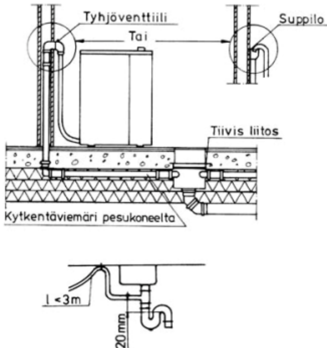
Kuva 29.1 Esimerkkejä kotitalouskäyttöön tarkoitetun pesu- tai astianpesukoneen viemärintitavoista.
