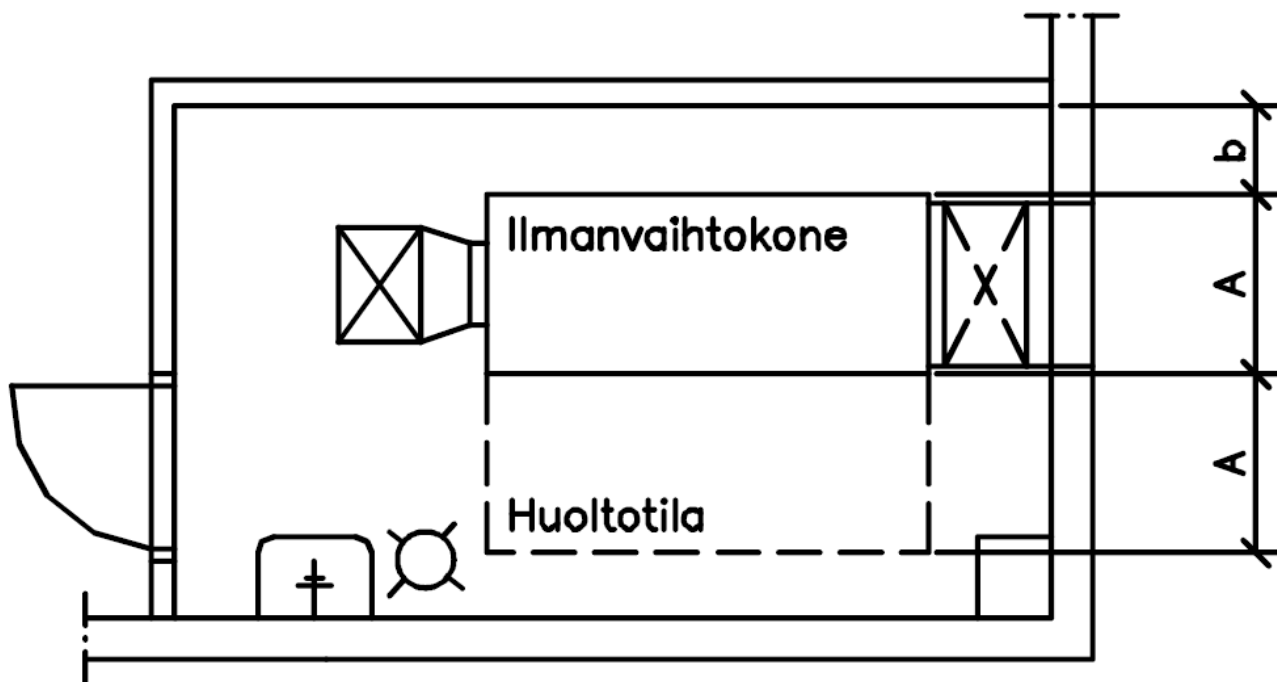
Kuva 24.1 Ilmanvaihtokoneen huoltotilan sijoitus- ja mitoitus esimerkki. A on ilmanvaihtokoneen leveys ja b on 0,4 kertaa ilmanvaihtokoneen korkeus tai vähintään 600 mm. Sijoitettaessa kaksi konetta samaan konehuoneeseen taustapuolelta vastakkain jätetään koneiden väliin huoltotilaksi sama etäisyys b.
