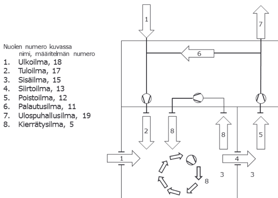
Kuva 1.1 Ilmavirtojen nimet ja määritelmät. Kuva on osittainen kopio standardin SFS-EN 16798-3:2017 standardista. Kuvaan on merkitty vain asetustekstin määritelmissä mainitut ilmavirrat.
