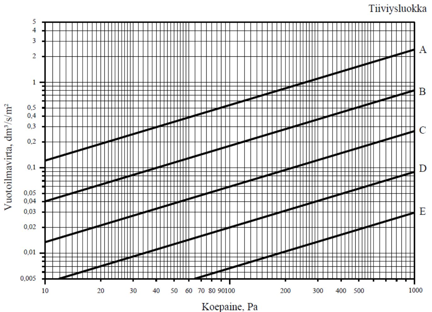
Kuva 19.1 Ilmanvaihtojärjestelmän ja sen osien suurimmat sallitut vuotoilmavirrat vaipan pinta-alaa kohti eri tiiviysluokissa.
