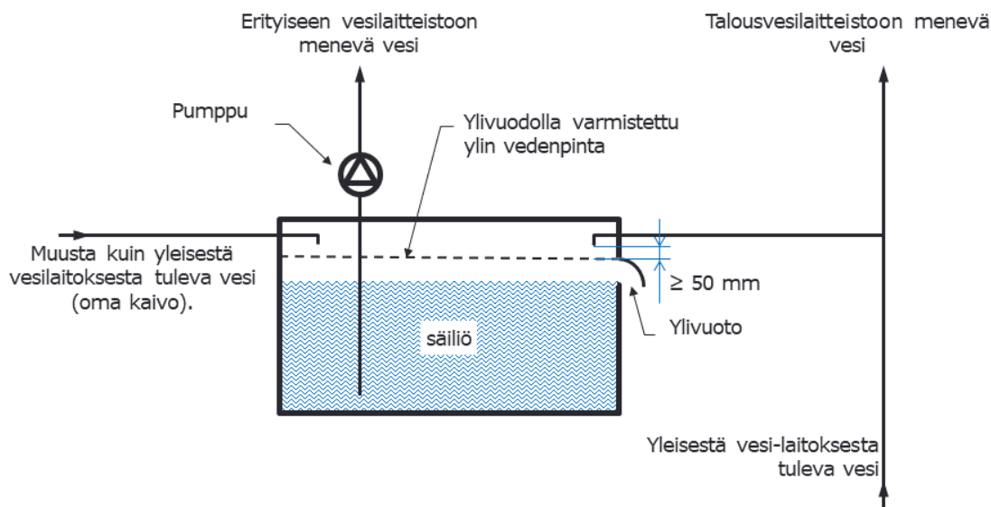
Kuva 5.1. Esimerkki veden johtamisesta vesihuoltolaitoksen verkosta ja muusta vesilähteestä käyttäen takaisinimusuojauksena AB.
