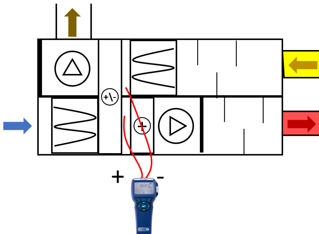
Kuva 61. Lämmöntalteenottokiekon paine-erojen mittaus [Antti Alanko]
