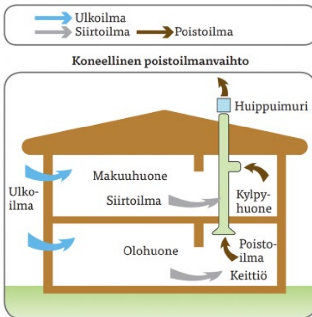
Kuva 1. Koneellinen poistoilmanvaihtojärjestelmä asuinrakennuksessa. [hengityslitto.fi]
