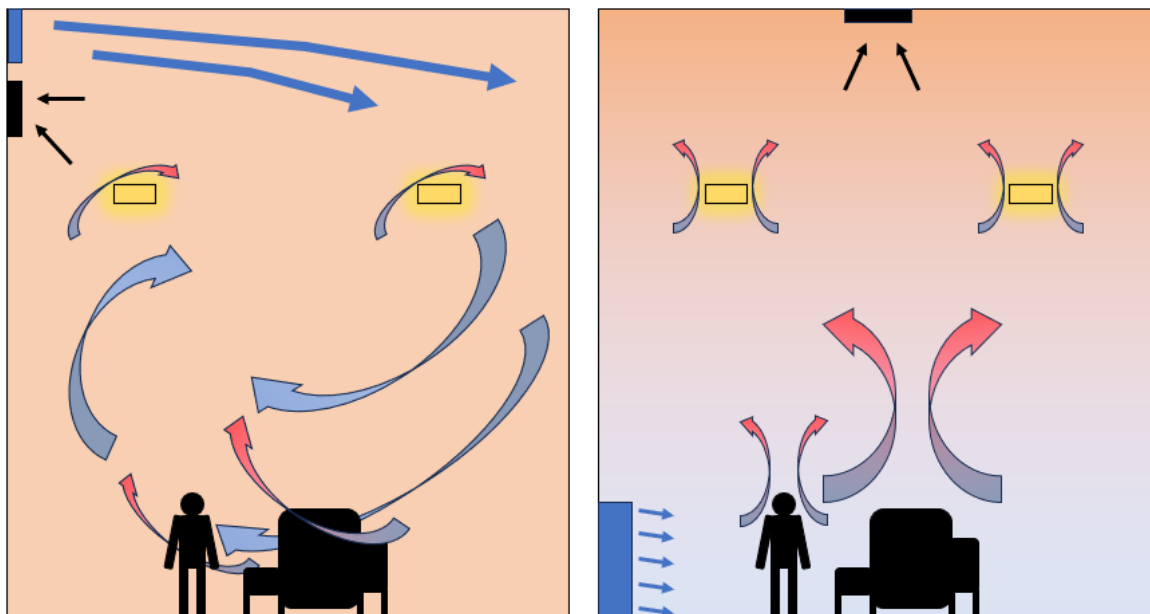
Kuva 6. Sekoittavan ja syrjäyttävän ilmanjaon periaatteet [Antti Alanko, mukaillen Kosonen, R. ym. 2014]
