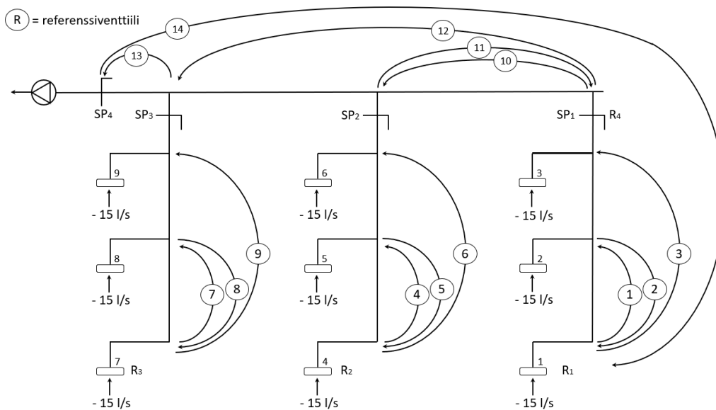
Kuva 64. Monihaaraisten ilmanvaihtojärjestelmän suhteellinen säätö. [Sami Mäkinen]
