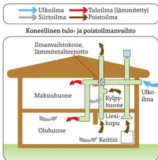
Kuva 3. Koneellinen tulo- ja poistoilmanvaihtojärjestelmä. [hengitysliitto.fi]
