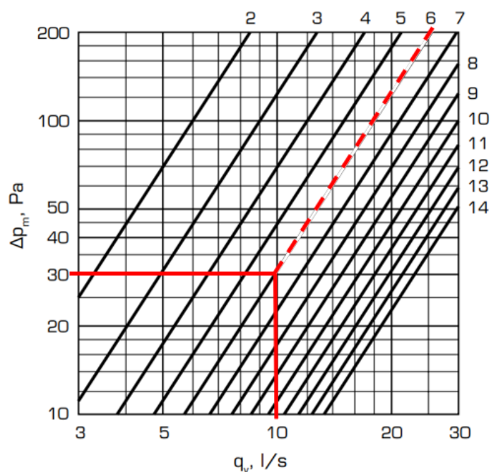
Kuva 46. Kun tiedämme paineen 30 Pa ja suunnitellun ilmavirran 10 l/s, säätökaavio kertoo, että venttiilin avaus pitää olla +6, jotta ilmavirta toteutuu. [FläktGroup säätöopas].
