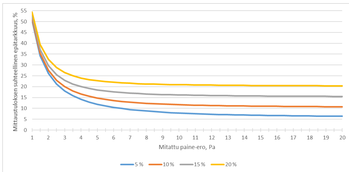
Kuva 44. Mittaustuloksen (l/s) suhteellinen epätarkkuus, kun mittarin tarkkuus on \pm 1 % lukemasta \pm 1 Pa, menetelmävirheen ollessa 5...20 % ja havaitsemisvirheen ollessa 5 %. [Antti Alanko]
