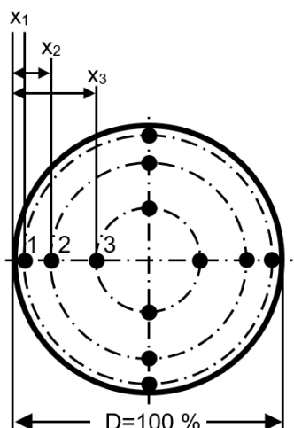
Kuva 54. Kanavamittauksen mittauspisteiden määrittäminen log-linear menetelmässä. Mittauspisteitä voi pienessä kanavassa olla 4, ja isommissa kanavissa mitattavia kehiä lisätään tarpeen mukaisesti. Taulukossa on esitetty mittauspisteen suhteellinen etäisyys kanavan sisäpinnasta, kun kehiä on 1...3 kpl (soveltaen SFS-EN 12599).
