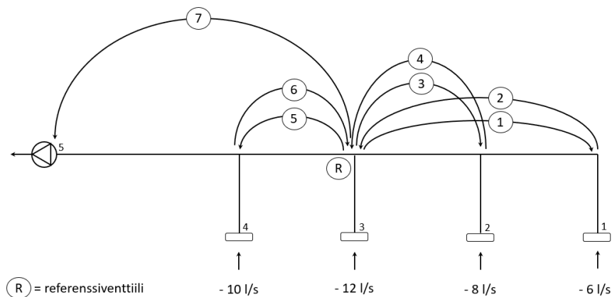
Kuva 63. Suhteellinen säätö, kun referenssilaitte ei ole linjan viimeinen päätelaite. [Sami Mäkinen]
