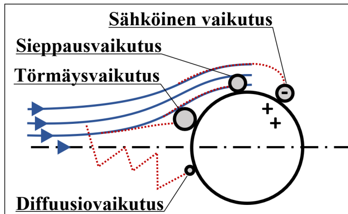
Kuva 12. Hiukassuodatuksen mekanismeja. Valkoinen ympyrä kuvaa suodattimen yksittäisen kuidun poikkileikkausta. [Antti Alanko, mukailen Koskinen, E. 2014]
