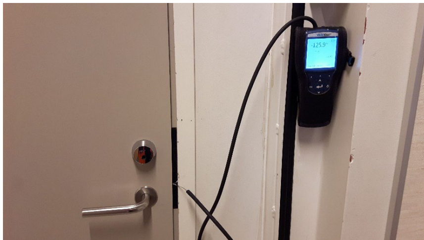
Kuva 59. Paine-eron mittaus kapillaarikoukulla välioiven yli [Antti Alanko]
