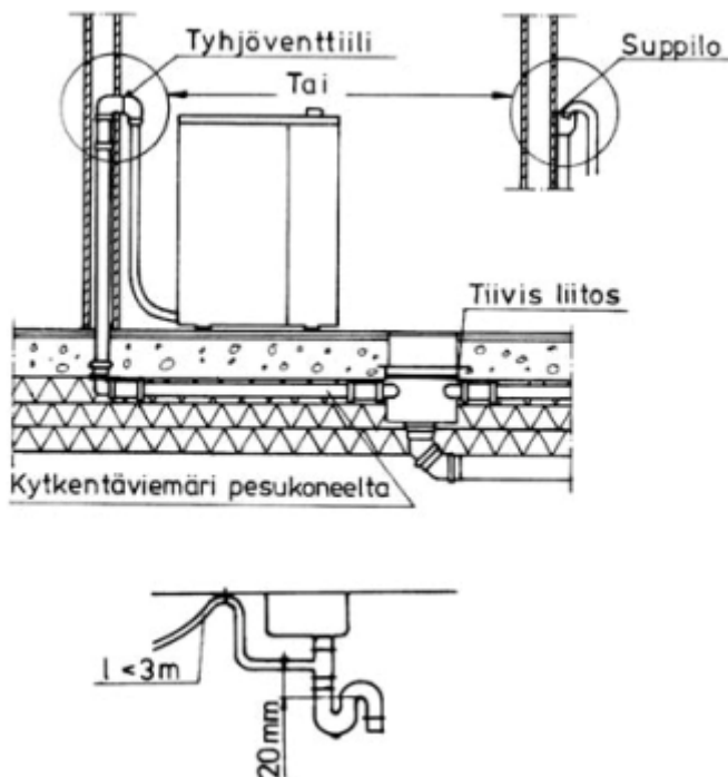
Kuva 29.1 Esimerkkejä kotitalouskäyttöön tarkoitettujen pesu- tai astianpesukoneiden viemärintavoista.
