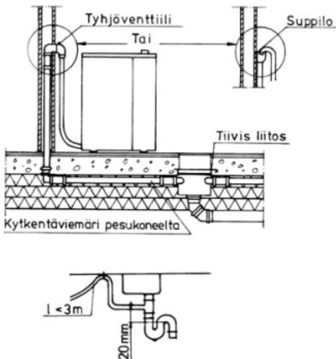
Kuva 29.1 Esimerkkejä kotitalouskäyttöön tarkoitettujen pesu- tai astianpesukoneiden viemärintäyttöistä.
